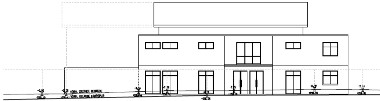
SÜDOST-ANSICHT
